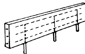
SW.025.3 (Für Rundungen geeignet) Mit Stahleinlage und Anker zum Einbetonieren in Betonfundament, Nutzungshöhe ca 25 cm 100 x 25 x 5 cm
