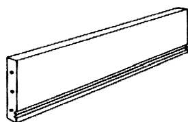
SW.025.1 Ohne Stahleinlage mit einseitigen Längsrillen zum Einbetonieren in Betonstütze, Nutzungshöhe ca 15 cm, 100 x 25 x 5 cm
