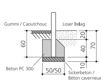
Pfosten einbetonieren / Sceller poteaux
