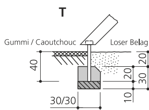
Treppe einbetonieren / Sceller escalier
