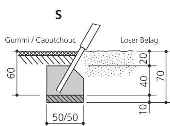
Pfosten einbetonieren Schrägnetz / Sceller poteaux filet oblique
