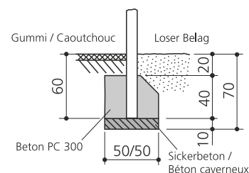
Pfosten einbetonieren / Sceller poteaux
