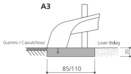
Spiralrutschbahn / toboggan en spirale
