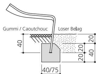
A1 Edelstahlrutschbahn / Toboggan en inox
