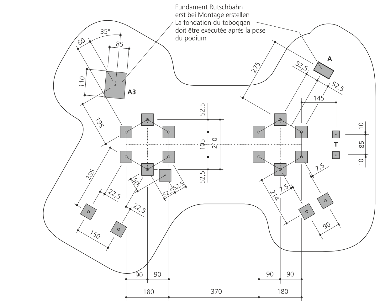
Spiralrutschbahn / toboggan en spirale
