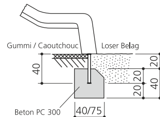
A2 Kunststoffrutschbahn / toboggan en polyester
