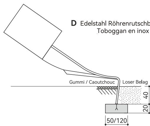
Pfosten einbetonieren / Sceller poteaux
