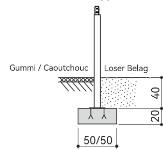
Pfosten C Edelstahl Röhrenrutschbahn / Poteau Toboggan en inox
