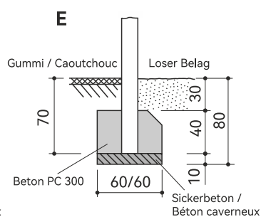
Pfosten einbetonieren / Sceller poteaux
