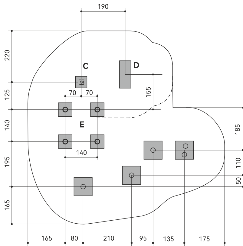
Pfosten C Edelstahl Röhrenrutschbahn / Poteau Toboggan en inox
