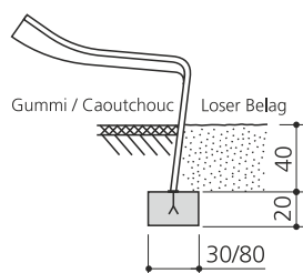
Kletterstange einbetonieren / Sceller perche à grimper
