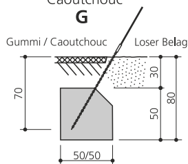
Schrägnetz einbetonieren / Sceller Filet oblique Fundament nachträglich / Fondation après montage Caoutchouc
