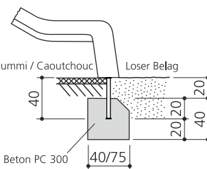
A2 Kunststoffrutschbahn / toboggan en polyester
