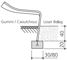
A1 Edelstahlrutschbahn / Toboggan en inox
