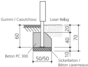
Pfosten einbetonieren / Sceller poteaux
