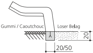
A2 Kunststoffrutschbahn / toboggan en polyester
