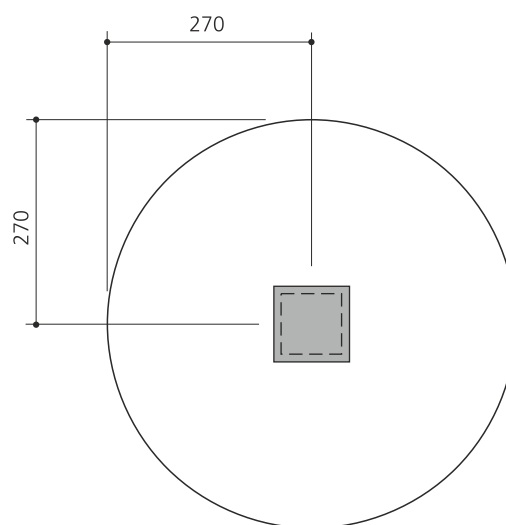
Fundament / Fondation
