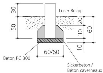
Pfosten einbetonieren / Sceller poteaux
