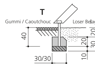
Treppe einbetonieren / Sceller escalier
