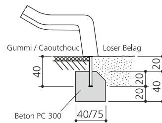
A2 Kunststoffrutschbahn / toboggan en polyester
