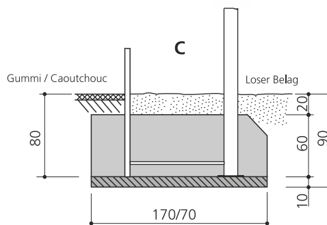
Pfosten und Kletterstange einbetonieren / Sceller poteaux et perche à grimper
