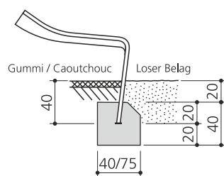
A1 Edelstahlrutschbahn / Toboggan en inox
