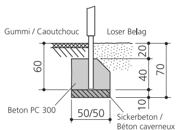
Pfosten einbetonieren / Sceller poteaux
