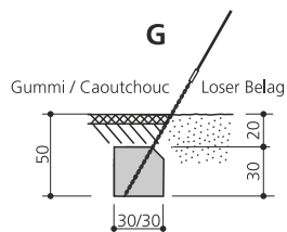
Schrägnetz einbetonieren / Sceller Filet oblique Fundament nachträglich / Fondation après montage Caoutchouc
