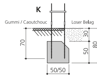
Strickleiter einbetonieren / Sceller échelle de corde Fundament nachträglich / Fondation après montage Caoutchouc
