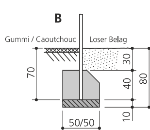
Kletterstange einbetonieren / Sceller perche à grimper
