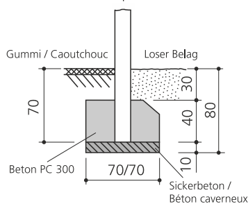
Pfosten einbetonieren / Sceller poteaux
