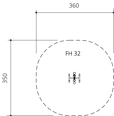
Grundriss / Plan
