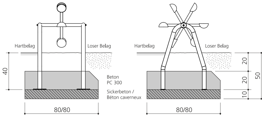
Pfosten einbetonieren / Sceller poteaux
