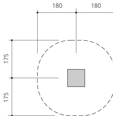
Fundamente / Fondations
